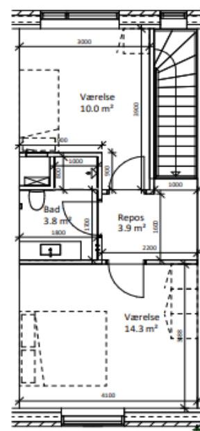
1. salsplan
